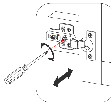
Horizontal adjustment Réglage horizontal Ajuste horizontal
